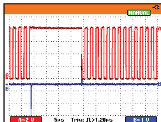
图 1. 在该 CMOS 设计中，一个 450 kHz 控制信号显示有不规则的中断。发现这种中断源自于复用器由于串扰的结果而在不正确的时间打开。红色轨迹(上)所示为具有中断的 450 kHz 信号。蓝色轨迹(下)所示为造成开关工作不正确的串扰。示波器在信号中断触发，该中断可看做是持续时间远远长于组成信号的脉冲的一个脉冲。450 kHz 方波的脉宽大约为 1.1 ms，因此选择触发设置为脉宽持续时间 > 1.2 ms，识别异常的脉冲。使用脉宽触发是将信号中断与主信号隔离的关键所在。
