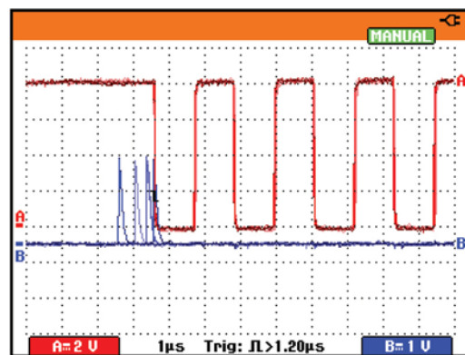
图 2. 当使用更高的时基速度时，能够明显看出串扰是由于一个未与 450 kHz 控制信号同步的子系统造成的。多亏有余辉模式，能够以类似于具有显示余辉的模拟示波器相似的方式显示连续的脉冲。
